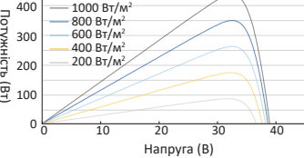
Крива «потужність-напруга» JAM54D41-440/LB
