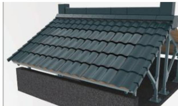
5-2-2.11 Установка боковой солнечной черепицы на крыше со стальной конструкцией, плоско-наклонной.
