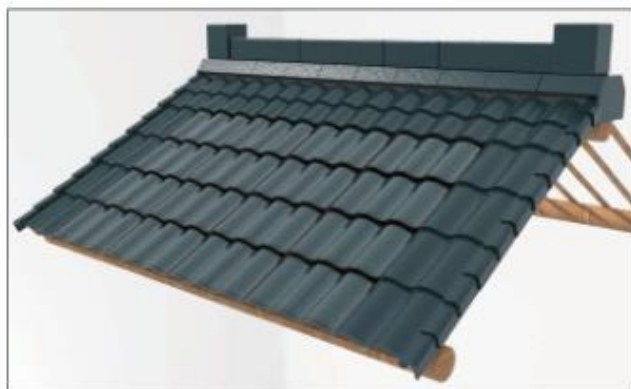
5.2.3.9 Установка боковой черепицы на крыше с деревянной конструкцией
